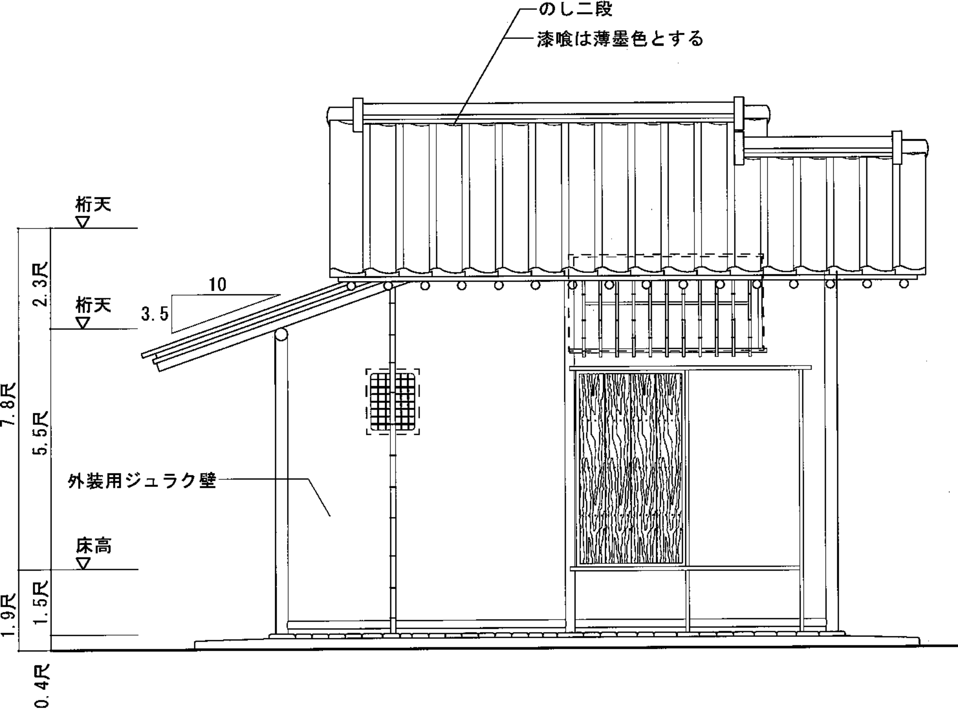
北側立面図 S=1:50
