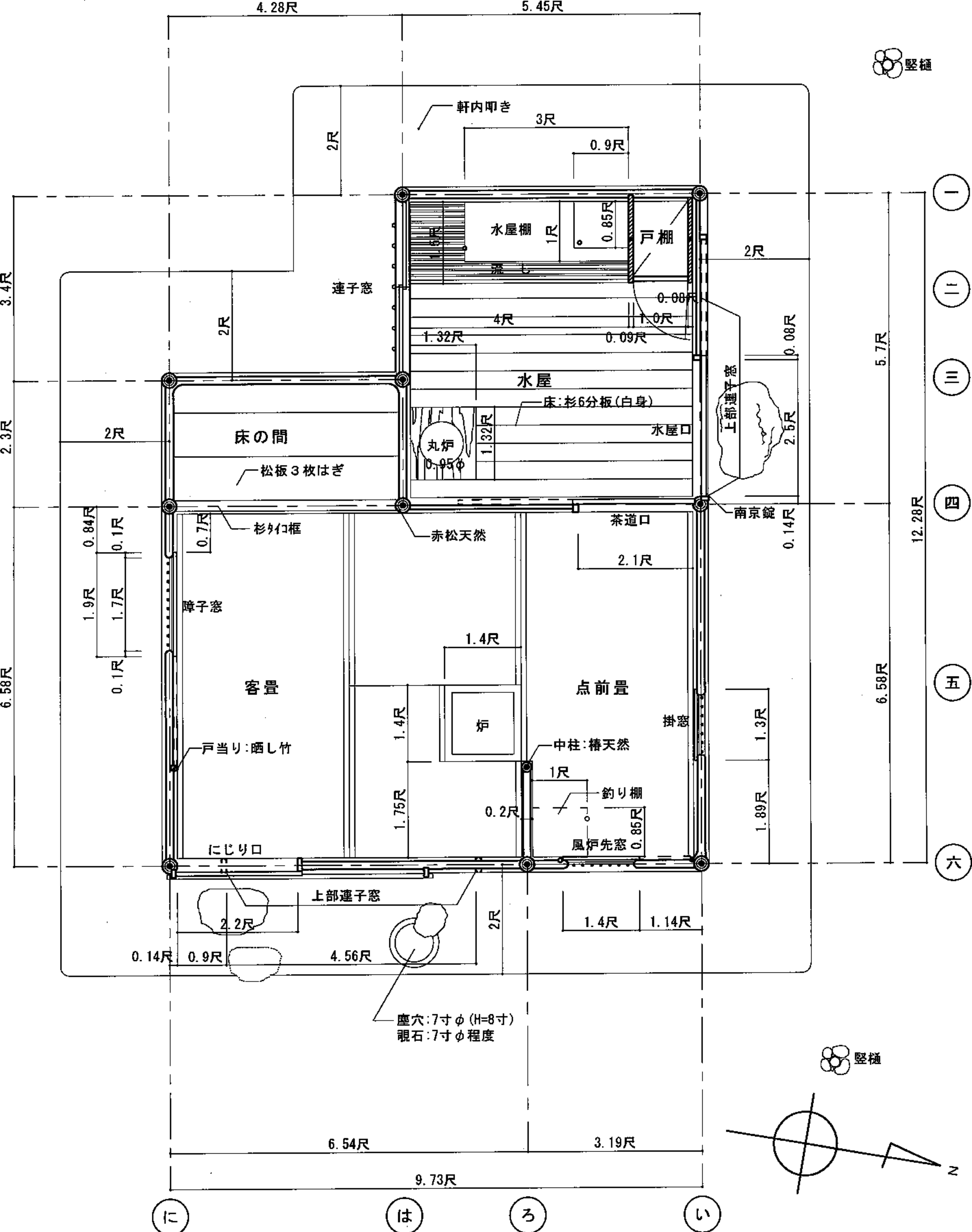
平面図 S=1:30
